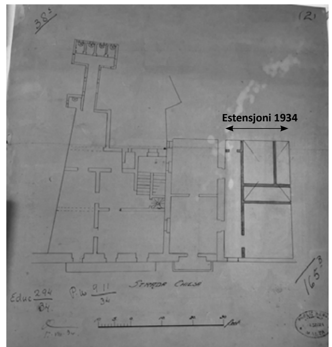
Figura 4a. Pjanta tal-ewwel pian tal-iskola fejn turi fejn ġejja l-estensjoni 12 .
