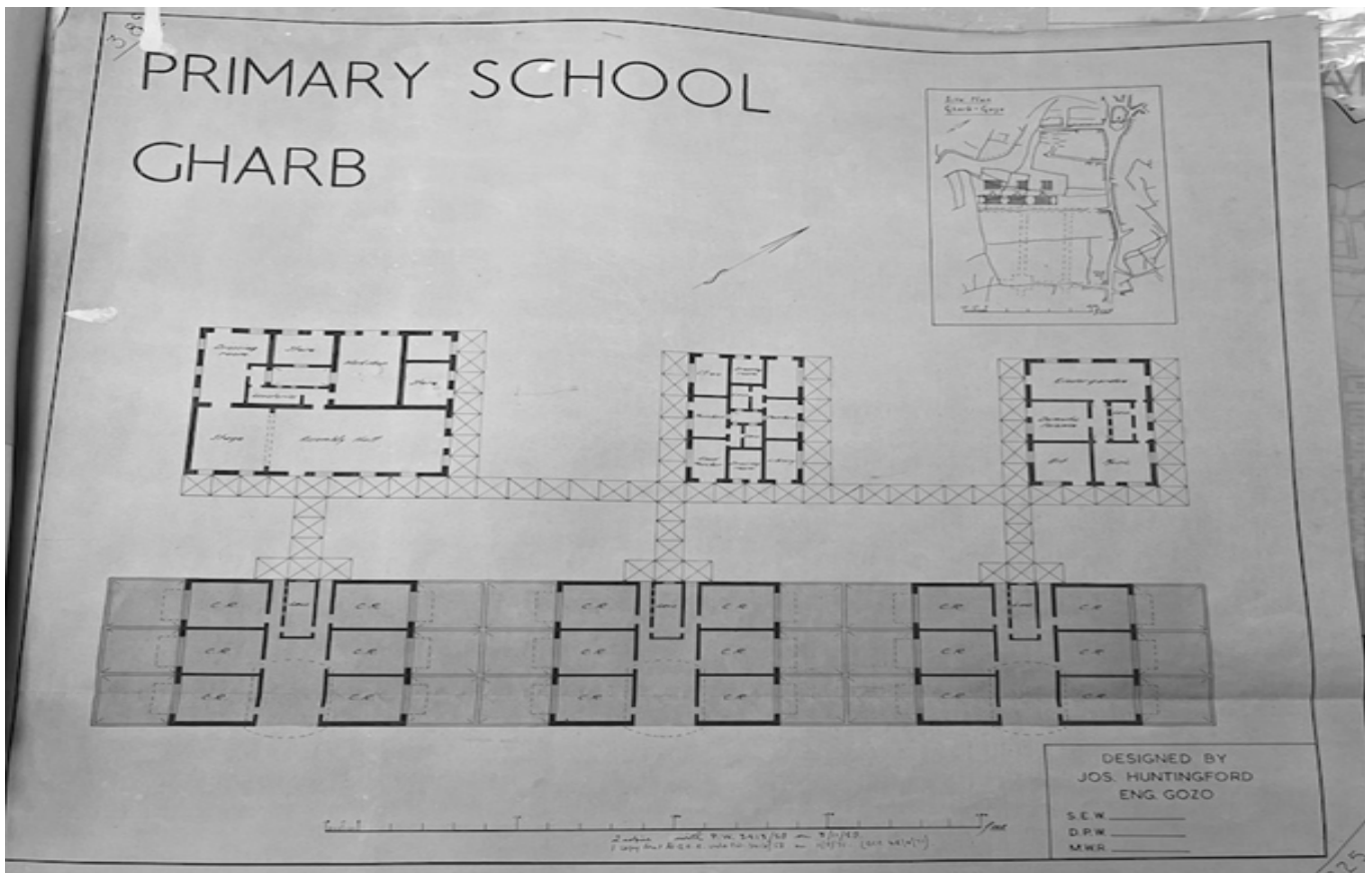
Figura 6. Pjanta tal-Iskola tal-Għarb iddisijata mil-Perit Joseph Huntingford 17 .
